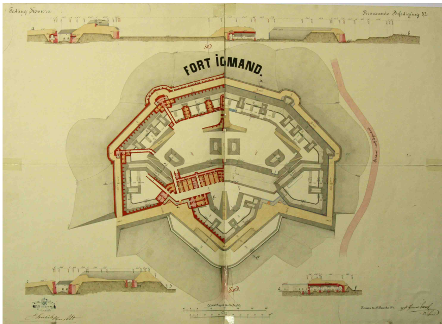
Igmándi erőd tervrajza
