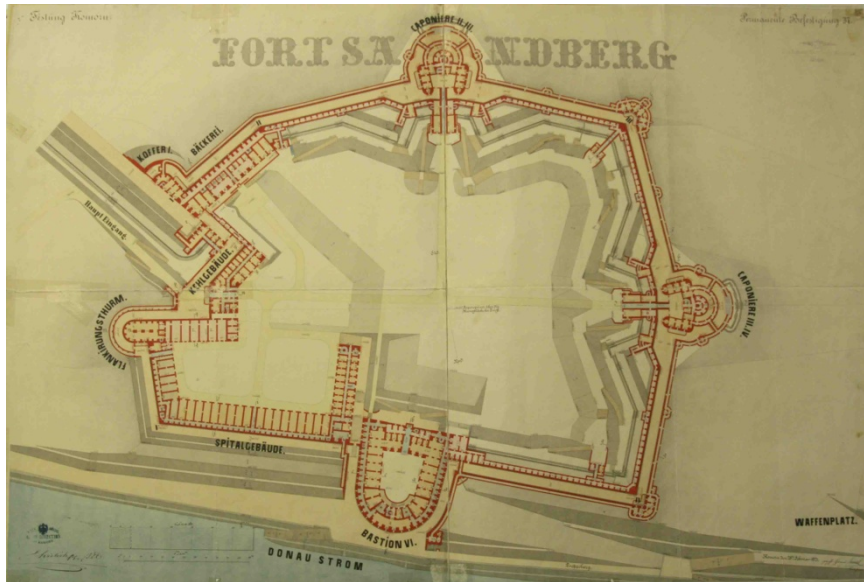
Monostori erőd tervrajza
